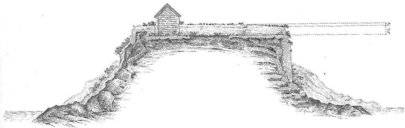
Corte por CD.
